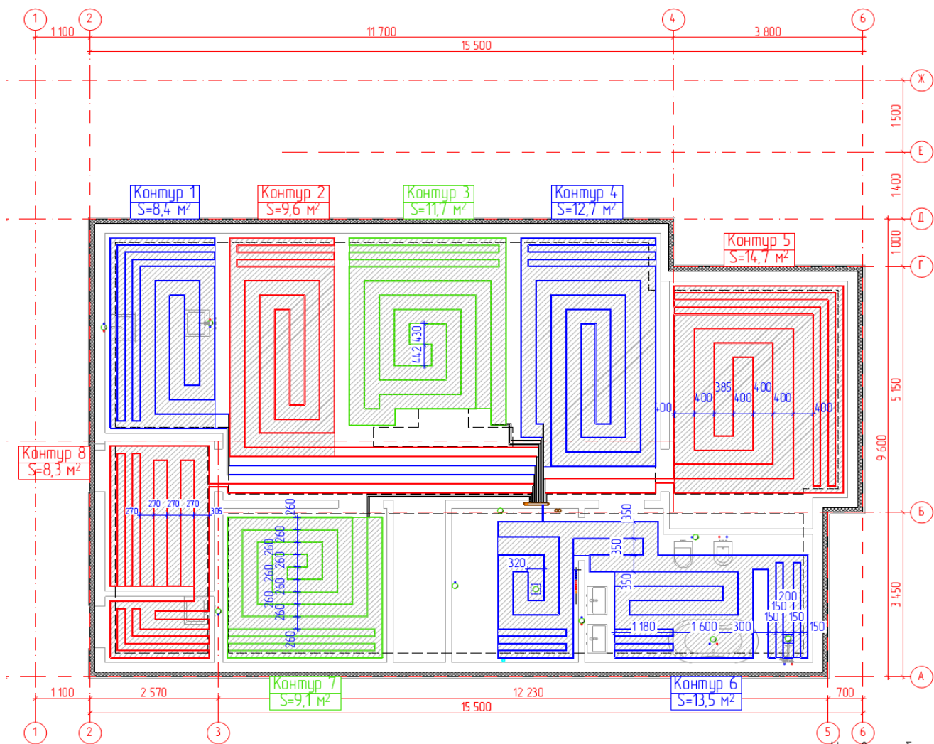
Схема расположения элементов водяного теплого пола. Схема намотки
