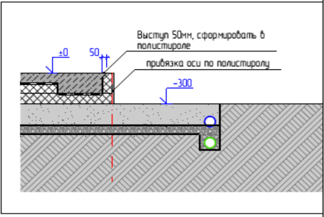
Схема устройства опалубки
